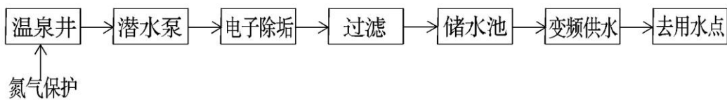
图 1-3 生产工艺流程图
