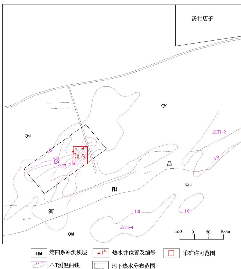
图 2-3 汤村汤地热田地温异常分布图
